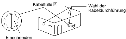
DETAIL ZUR DURCHFÜHRUNG DES VERBINDUNGSKABELS
