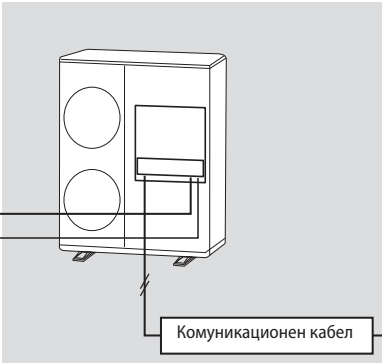
Външно тяло
