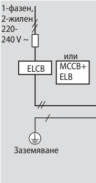
Разпределително табло
