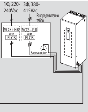
Хидроустройство
