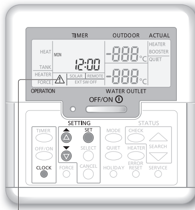
Indicador de Cuidado (Temperatura do depósito acima dos 60 °C)
