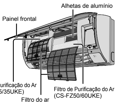
Filtro do ar
