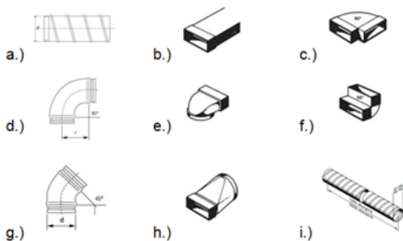
Fig. 6: Skematisk fremstilling af basiselementerne i et rørsystem til indsugning og udblæsning af luft
