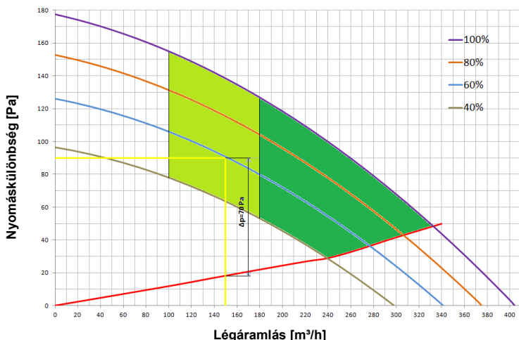
3. diagram: Példa az aerodinamikai jellemzők meghatározására
