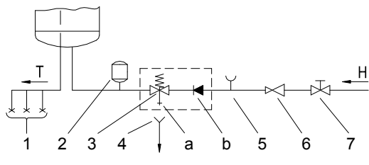
Fig. 7: Stängt (tryck-)system
