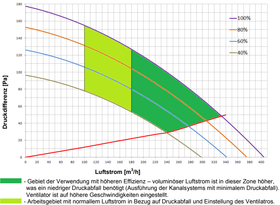
Graf 1: Aerodynamische Charakteristiken
