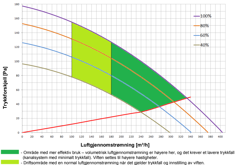
Diagram 1: Aerodynamiske egenskaper
