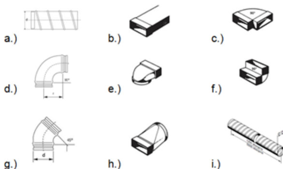
Rysunek 6: Schemat podstawowych elementów systemu rurociągowego dla doprowadzenia i odprowadzania powietrza
