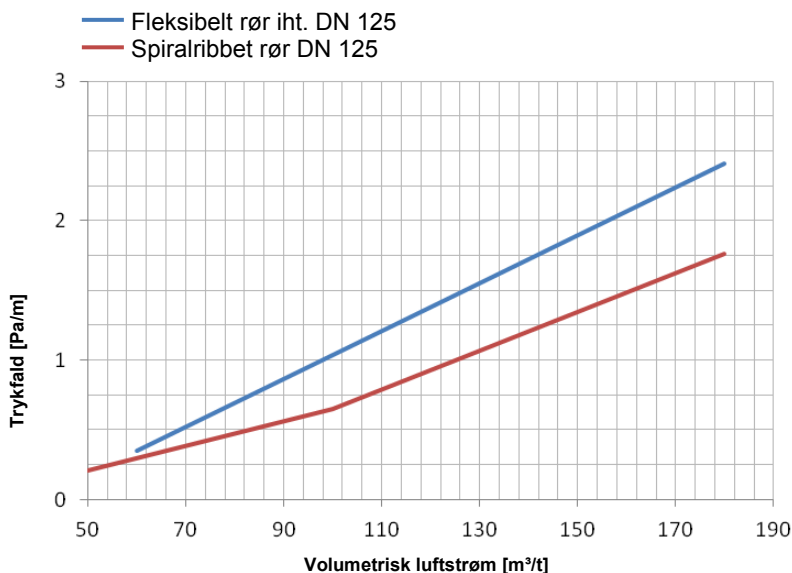
Diagram 2: Værdi af det statiske trykfald for de valgte rør
