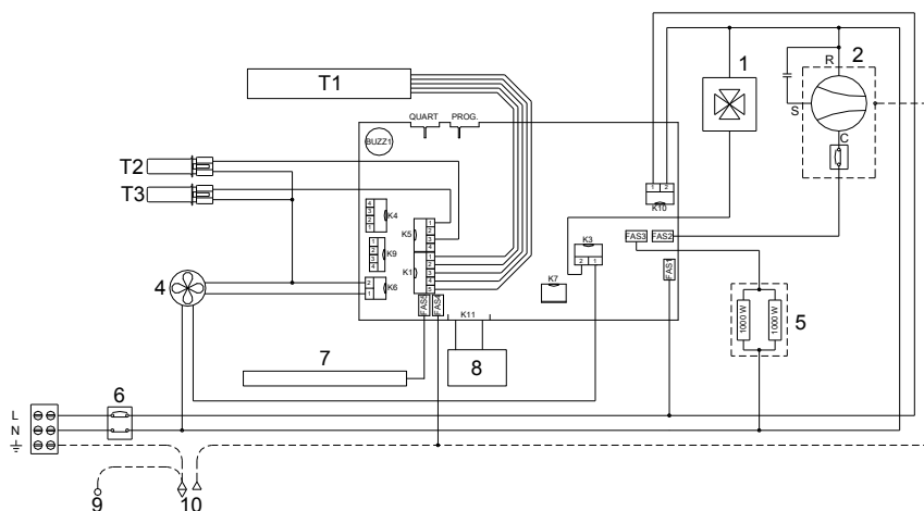
Fig. 10: El-diagram
