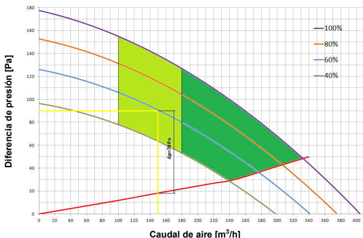
Gráfico 3: Ejemplo de determinación de la característica aerodinámica
