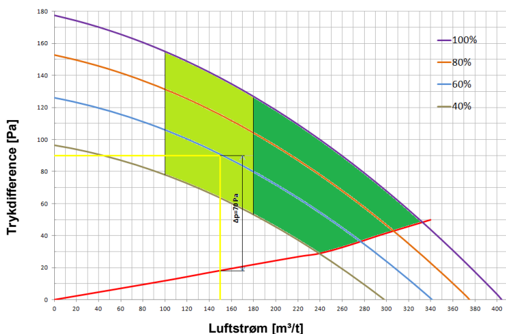
Diagram 3: Eksempel på bestemmelse af aerodynamisk egenskab
