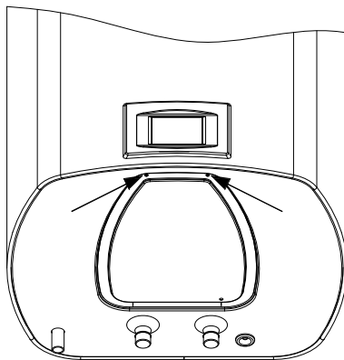
9. ábra: Védőfedél
