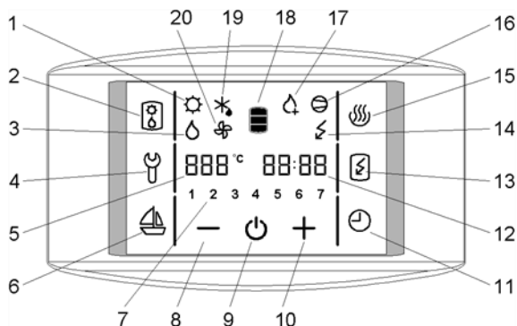
Fig.11: LCD-touchskærm
