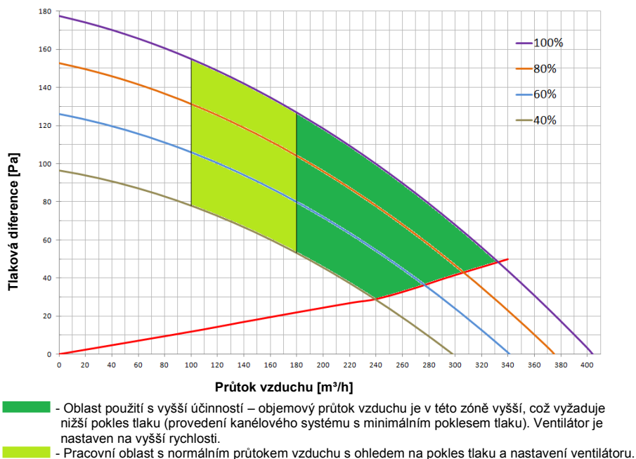
Graf 1: Aerodynamické charakteristiky
