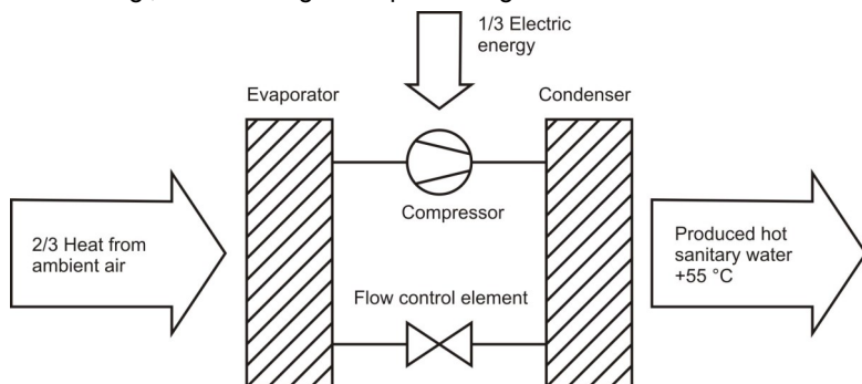
Fig. 1: Diagram over energiflowet gennem varmepumpeenheten
