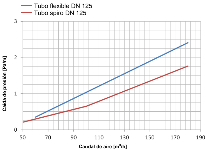
Gráfico 2: Valor de la caída de presión estática para diferentes tubos
