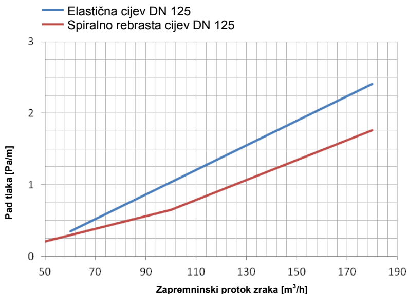
Grafikon 2: Vrijednost pada statičnoga tlaka za odabranu cijev
