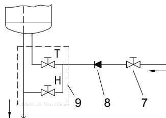
8. ábra: Nyitott (nem nyomásos) rendszer
