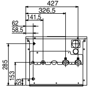
ALTITAN GÖRÜNÜM
