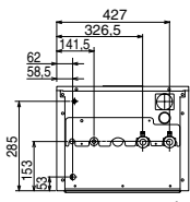
BILD UNDERIFRÅN
