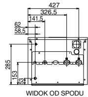
WIDOK OD SPÓDU
