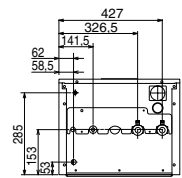
SETT FRA UNDERSIDEN
