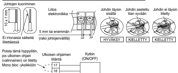
Taulukko 4,2: Ulkoinen ohjaimen liitäntäkaavio
