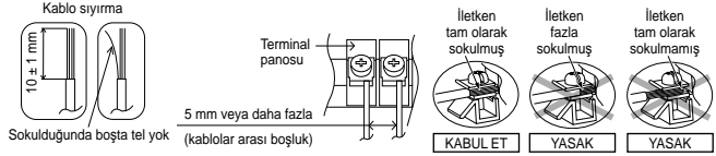
Şema 4.2: Harici Kontrol Ünitesi bağlantı şeması
