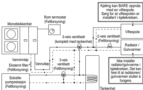
Tegning 3,1: Typisk installasjon av vannrør
