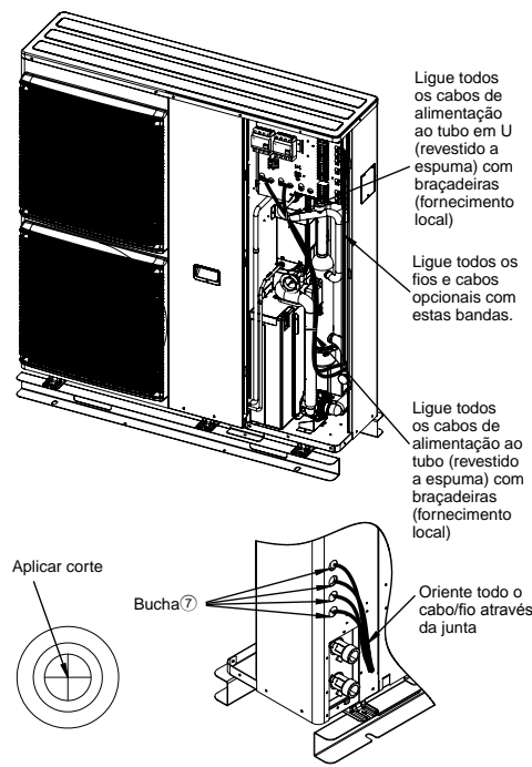
Como orientar o cabo / fio com as buchas
