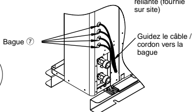
Comment guider le câble / cordon vers la bague
