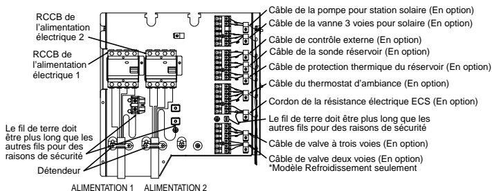
Comment guider les cordons d'alimentation et le câble / cordon optionnel (Vue sans câblage interne)
