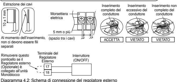
Diagramma 4,2: Schema di connessione del regolatore esterno
