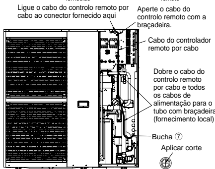
Como ligar o controlo remoto ao conector fornecido
