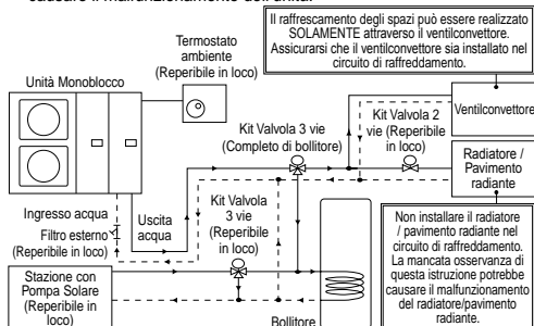
Diagramma 3.1: Installazione tipica dei tubi dell'acqua
