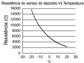
Gráfico 4,1: Característica do sensor do depósito
