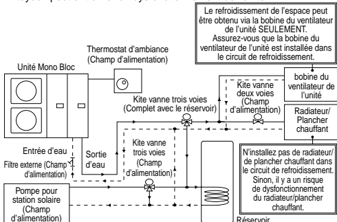
Schéma 3.1 : Installation de tuyauterie d'eau typique
