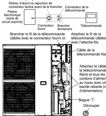
Comment connecter la télécommande au connecteur fourni
