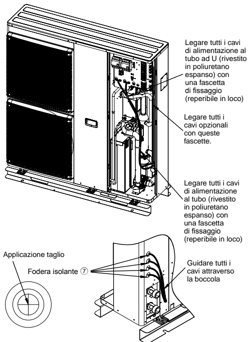
Come guidare il filo / cavo sulla fodera isolante
