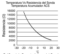
Gráfico 4.1: Características de la Sonda Temperatura Acumulador ACS
