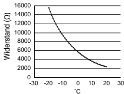
Abbildung 4.1: Kennlinie des Speichertemperaturfühlers
