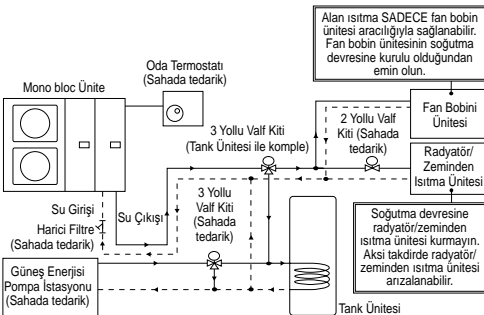
Şema 3.1: Tipik Su Boru Tesisatı
