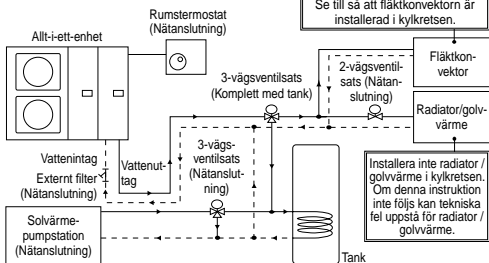
Diagram 3.1: Typisk vattenledningsinstallation
