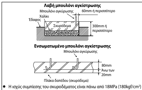
Εικόνα τύπου λαβής και τύπου ενσωματωμένου μπουλονιού ακιρώσεως
