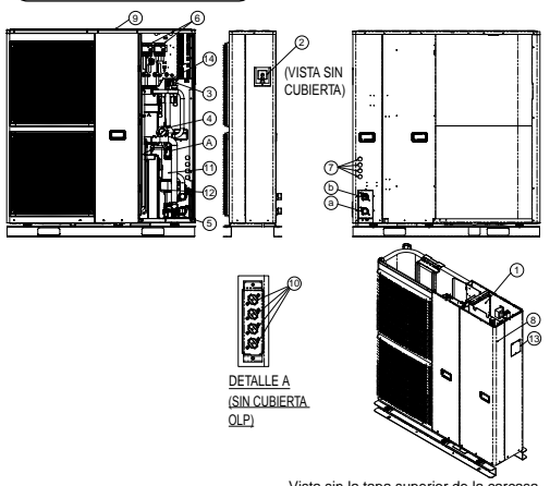
Vista sin la tapa superior de la carcasa
