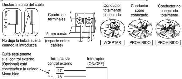
Diagrama 4.2: Diagrama de conexión de control externo
