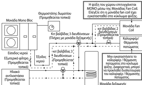
Διάγραμμα 3,1: Τυπική εγκατάσταση σωλήνωσης νερού
