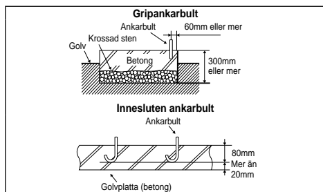
Bild på ankarbult av griptyp och innesluten typ
