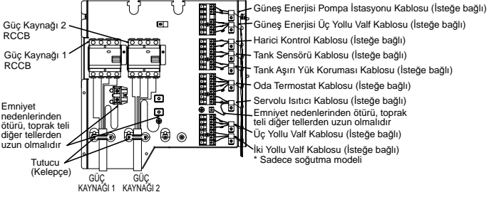
Güç kaynağı kablolarının ve isteğe bağlı kablounun yönlendirilmesi (Dahili kablolama olmadan görünüm)
