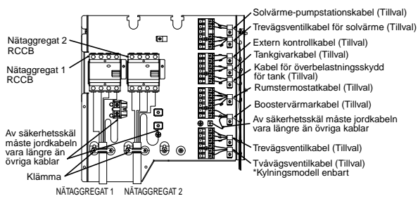
Hur du leder nätkablar och tillvalskabel/-sladd (vy utan intern kabeldragning)
