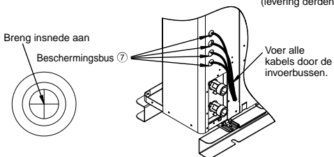
Hoe de Kabel/het snoer naar de doorvoer te leiden
