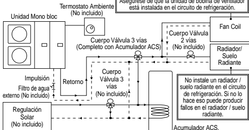
Diagrama 3.1: Instalación de tubería de agua típica
