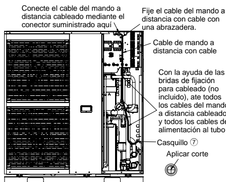
Cómo conectar el mando a distancia al conector suministrado
