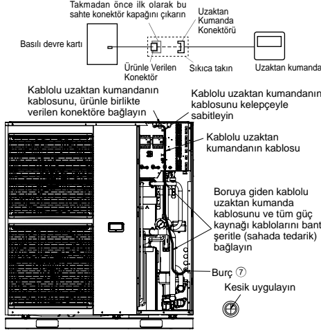
Uzaktan Kumandanın Ünite Verilen Konektöre Bağlanması
