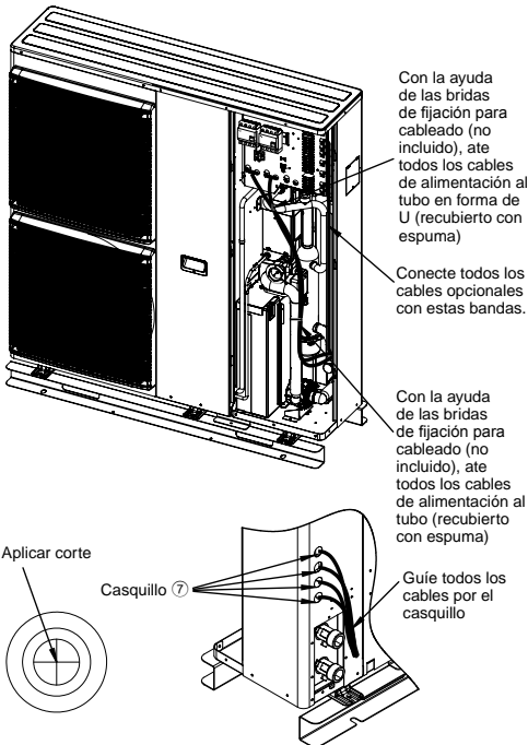
Como guiar cables por el casquillo
