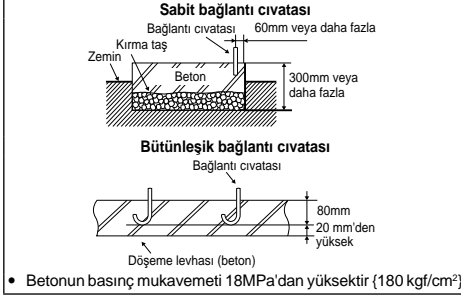
Sabit tip ve bütünlük tip bağlantı civatası çizimi
