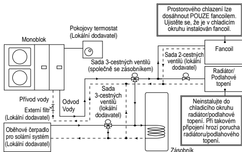
Diagram 3.1: Typická instalace vodního potrubí
