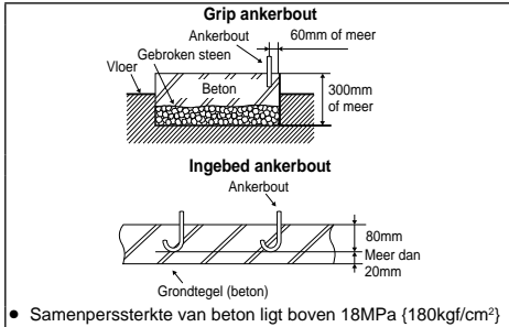
Abbeelding van de ankerbout van het type met greep en het inbouwtype
