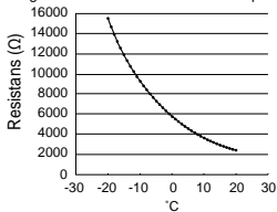
Graf 4.1: Tankgivarregenskaper
