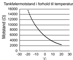
Figur 4,1: Tankfølerkarakteristikk
