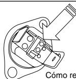
Cómo reiniciar el Klixon seguridad (10)
