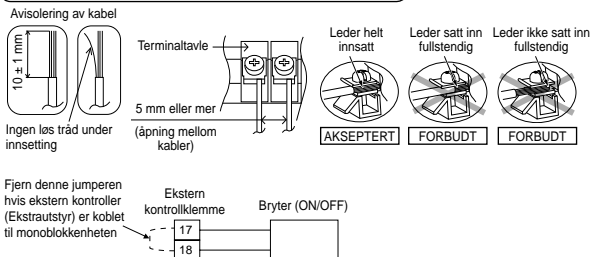
Tegning 4,2: Ekstern kontroll tilkoblingskjema
