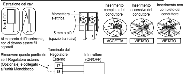
Diagramma 4,2: Schema di connessione del regolatore esterno
