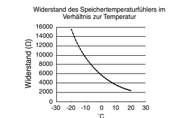
Abbildung 4.1: Kennlinie des Speichertemperaturfühlers
