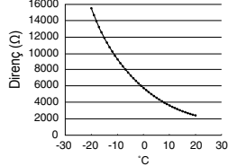
Grafik 4.1: Tank sensörü karakteristik özellikleri
