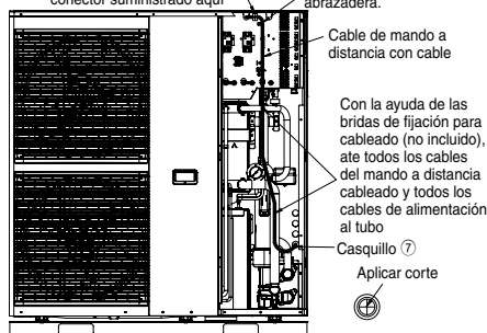
Cómo conectar el mando a distancia al conector suministrado
