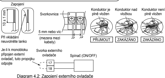
Diagram 4.2: Zapojení externího ovladače
