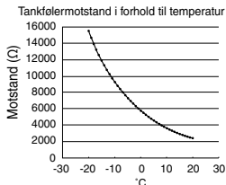
Figur 4,1: Tankfølerkaraktistikk
