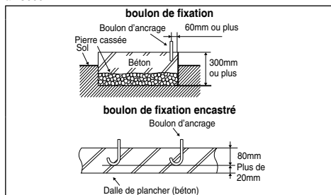
Illustration du boulon d'ancrage de type grippant et de type encastré
