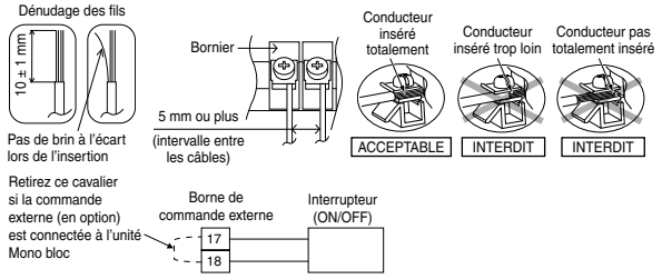
Schéma 4.2 : Schéma de raccordement de la commande externe
