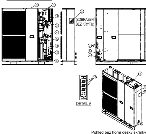
Pohled bez horní desky skříňky
