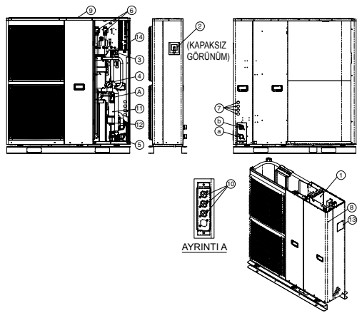
Dolap üst plakası olmadan görünüm
