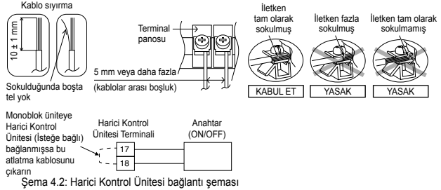
Şema 4.2: Harici Kontrol Ünitesi bağlantı şeması
