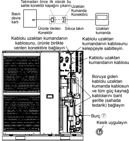
Uzaktan Kumandanın Üniteye Verilen Konektöre Bağlanması
