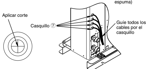
Como guiar cables por el casquillo
