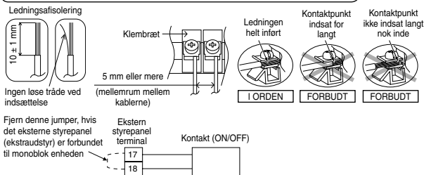
Diagram 4.2: Forbindelsesdiagram for ekstern styrepanel kabel
