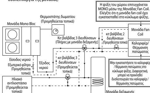
Διάγραμμα 3.1: Τυπική εγκατάσταση σωληνώσεων νερού
