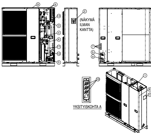
Näkymä ilman kotelon yläkantta
