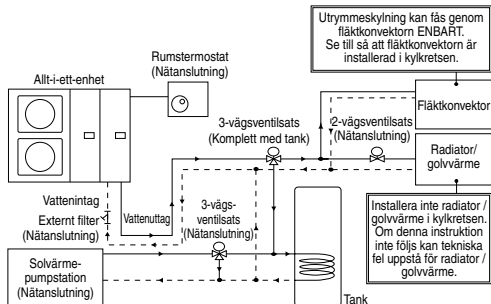
Diagram 3.1: Typisk vattenledningsinstallation
