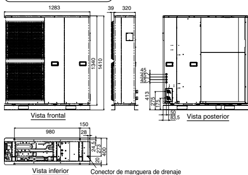
Conector de manguera de drenaje
