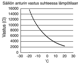
Käyrä 4,1: Säiliön anturin määritykset
