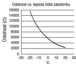
Graf 4.1: Popis čidla zásobníku
