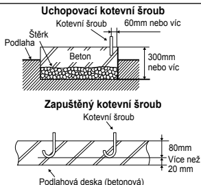
Nákres uchycení a zapuštěných kotevních šroubů
