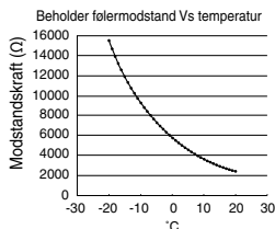
Graf 4,1: Beholder følger egenskaber
