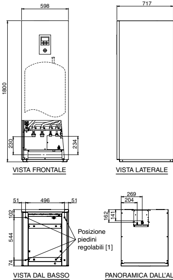
Diagramma delle dimensioni
