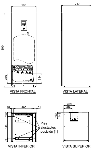
Diagrama de dimensiones
