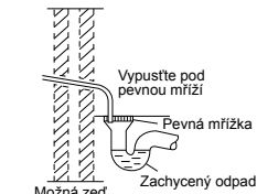
Zobrazení vodící hadice kondenzátu do venkovních prostor
