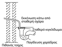
Εικόνα δρομολόγησης σωλήνα αποσπράγγισης προς το εξωτερικό
