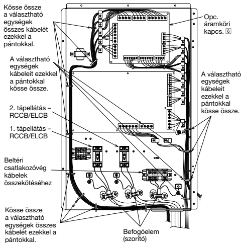
A választható kábelek és a tápkábel vezetésének módja (belső vezetékezés nélküli nézet)
