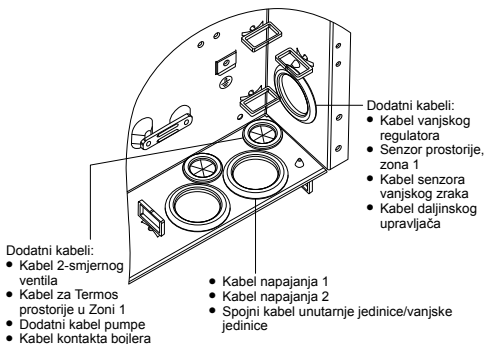
Usmjeravanje dodatnih kabela i kabela napajanja (prikaz bez internog ožičenja)
