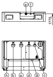
Diagrama de posición de tubo
