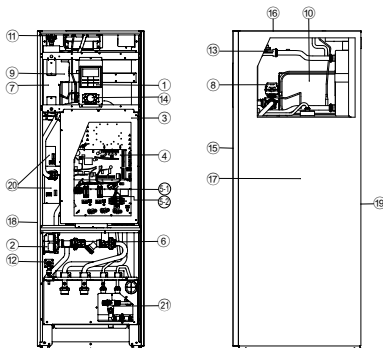
Diagrama de componentes principales
