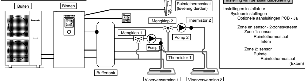
Vloerverwarming 1 + Vloerverwarming 2
