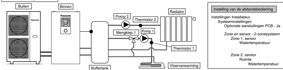
Vloerverwarming + Radiator
